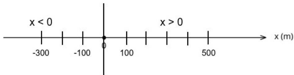
Figura 3: Criterio de signos de posición
