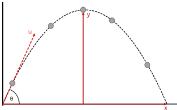
Figura 6: Trayectoria curva de una pelota al tirar a canasta
